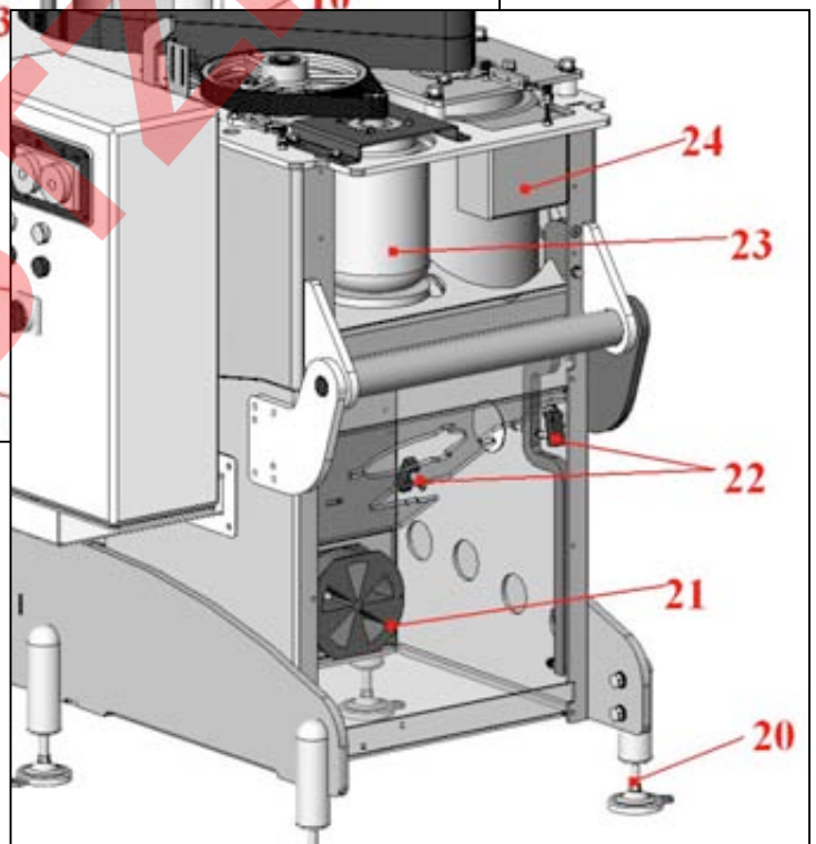
IMPASTATRICI A VASCA ESTRAIBILE VE-80
